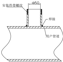
插入式电磁流量计现场带压、带水安装步骤示意图
