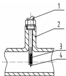
图 18 直面管道的插入方式
