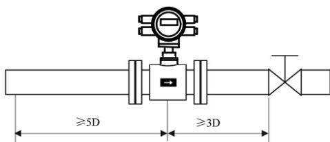
图 8 阀门位于传感器下游的安装
