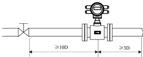
图 9 阀门位于传感器上游的安装
