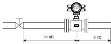
阀门位于传感器上游的安装
