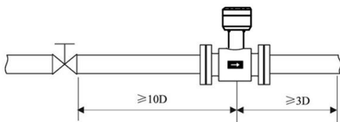
图 7 阀门位于传感器上游的安装
